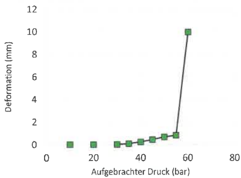
Sonde 3 (Schrägzugversuch), vertikale Deformation
