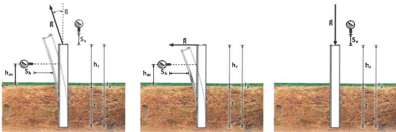
Schematische Darstellung durchgeführter Probekbelastungen (von links nach rechts): Schrägzugversuch, Horizontalversuch (ebenfalls Zug) und Druckversuch. Zeichenerklärung: R [kN] - Zugkraft, \beta [°] - Kraftansatzwinkel, h_m [m] - Kraftansatzhöhe, l_p [m] - gesamte (wirksame) Länge, t [m] - Einbindetiefe des Rammprofils, s_h [mm] - Verformung horizontal, s_v [mm] - Verformung vertikal. Die Instrumentierung der Probepfähle erfüllt die grundsätzliche Anforderungsstufe (EA Pfähle, 9.2.2.4). Der axiale Druckversuch (Bild 3) wird mittels Rammsondierung oder Handpenetrometer abgeschätzt.
