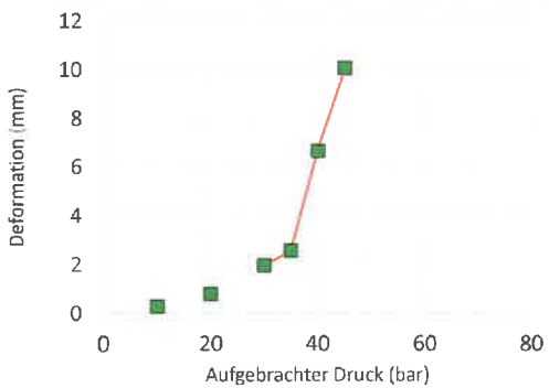
Sonde 7 (Schrägzugversuch), vertikale Deformation
