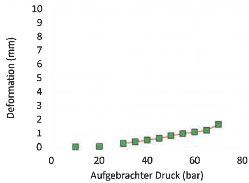
Sonde 4 (Schrägzugversuch), vertikale Deformation
