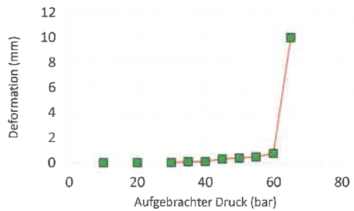
Sonde 22 (Schrägzugversuch), vertikale Deformation
