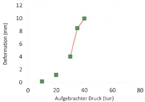
Sonde 8 (Schrägzugversuch), vertikale Deformation
