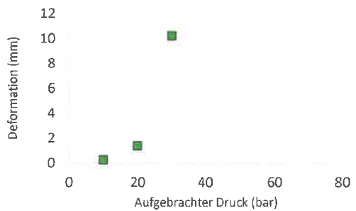
Sonde 24 (Schrägzugversuch), vertikale Deformation
