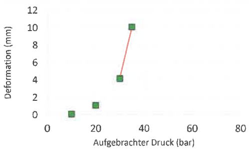
Sonde 23 (Schrägzugversuch), vertikale Deformation
