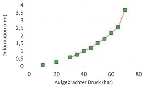
Sonde 21 (Schrägzugversuch), vertikale Deformation
